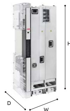
ACS880-14/34 R11
